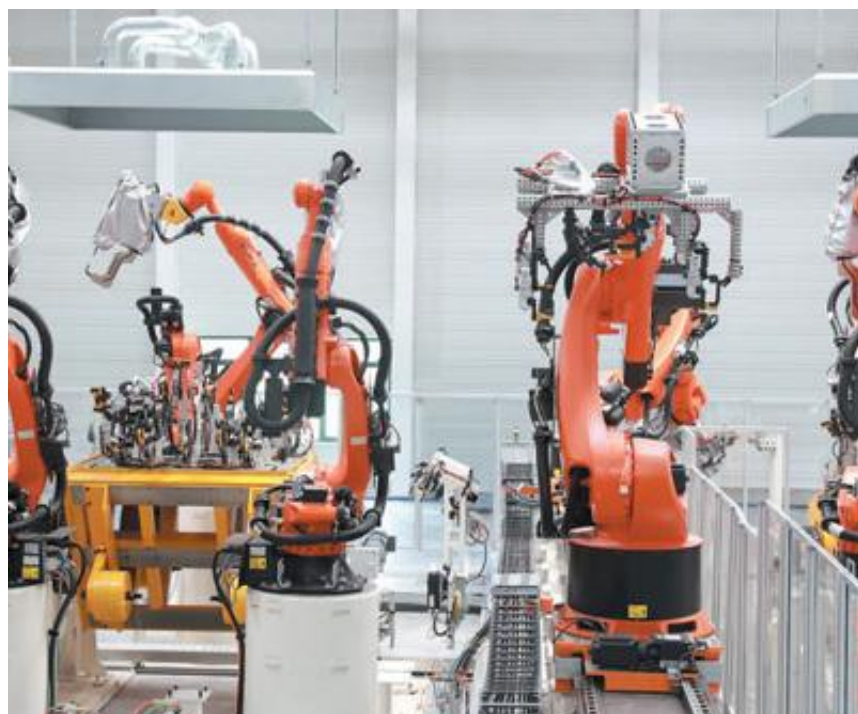
大众安徽新能源汽车工厂车身车间。图为受访企业提供
